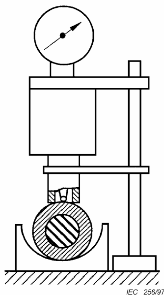
Figure C.2a – Eprouvette dans une goulotte
